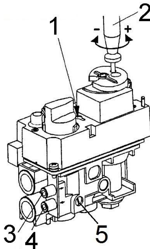
Abb. 8: Gasregelblock
